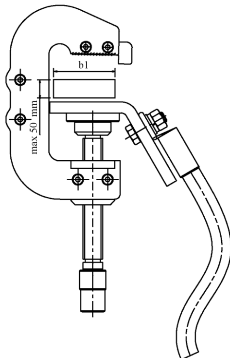
Zacisk uziomowy WZ-1
